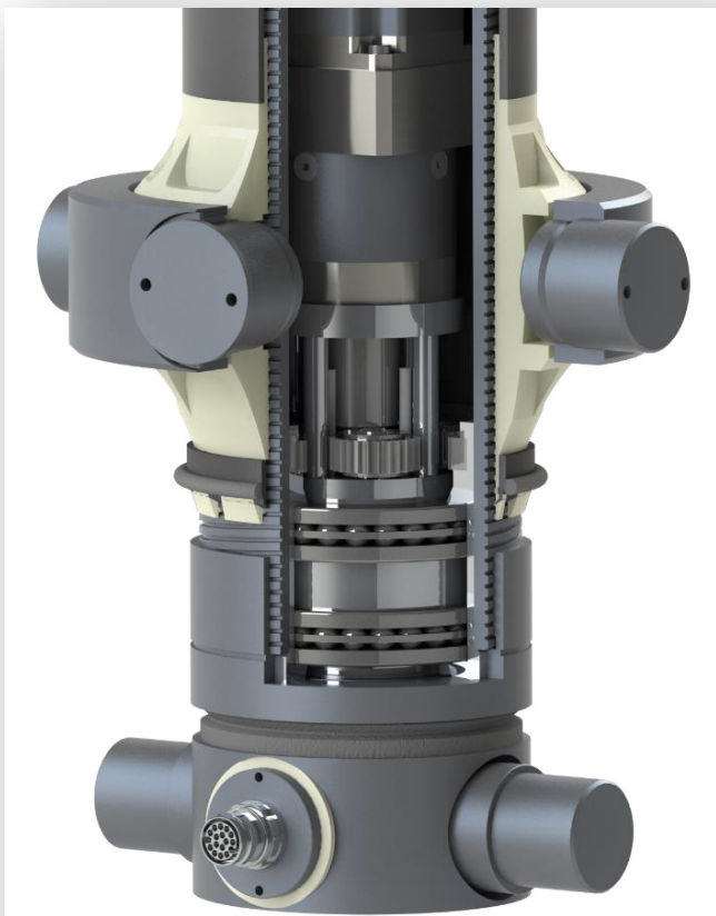
Innenliegender Spindelantrieb mit kreuzkardanischer Aufhängung Inside screw drive with cross-cardanic suspension
