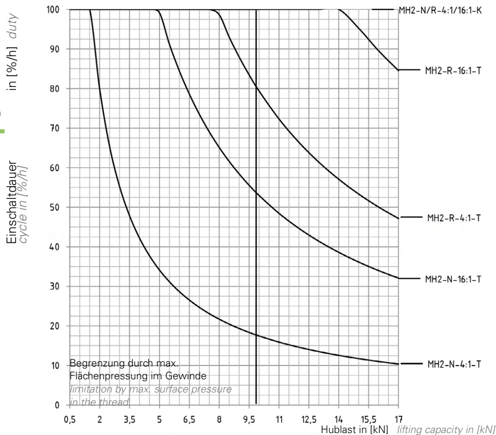
Einschaltdauerdiagramm MH2 duty cycle diagram MH2
