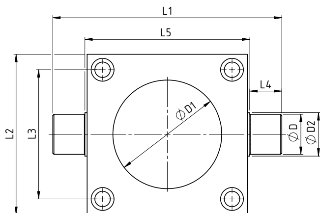
Darstellung für Ausführung KA-G2. Illustration for version KA-G2.
