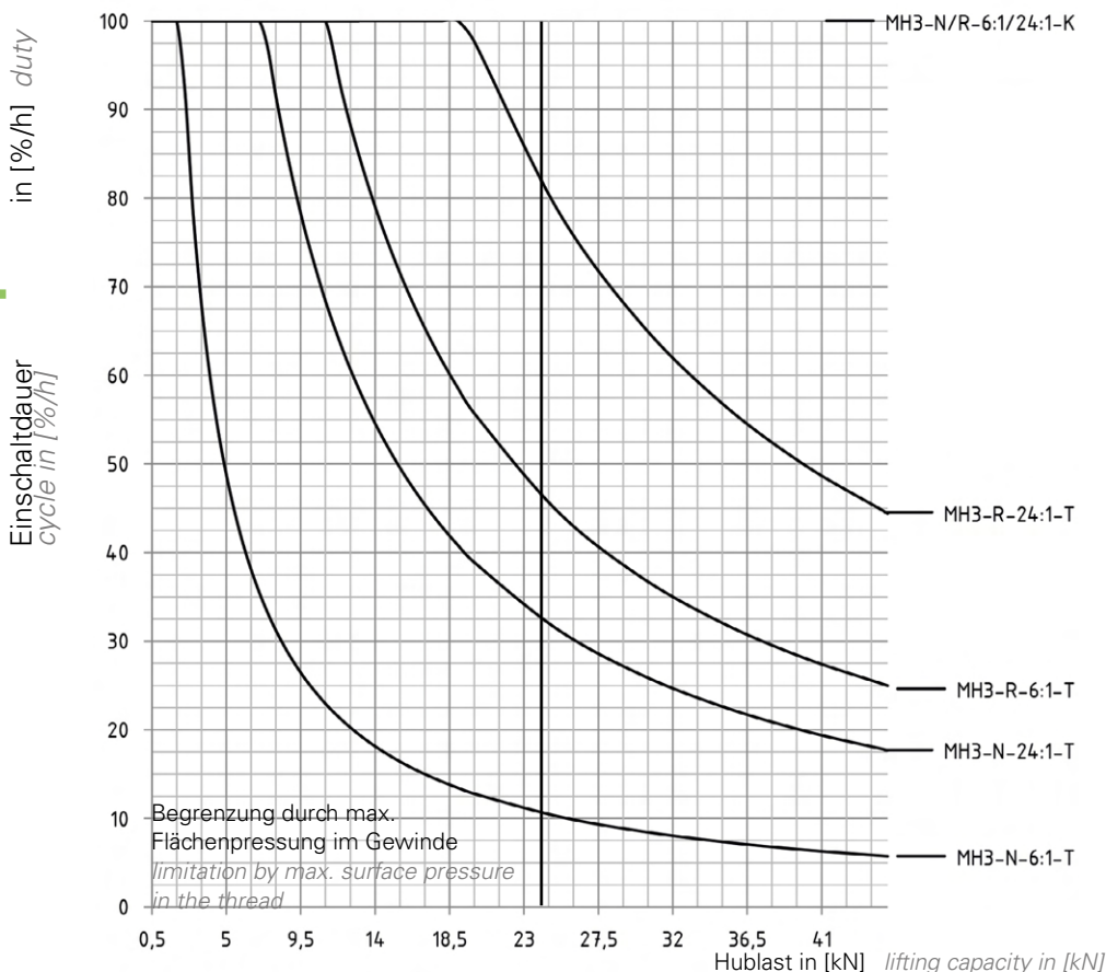
Einschaltdauerdiagramm MH3 duty cycle diagram MH3
