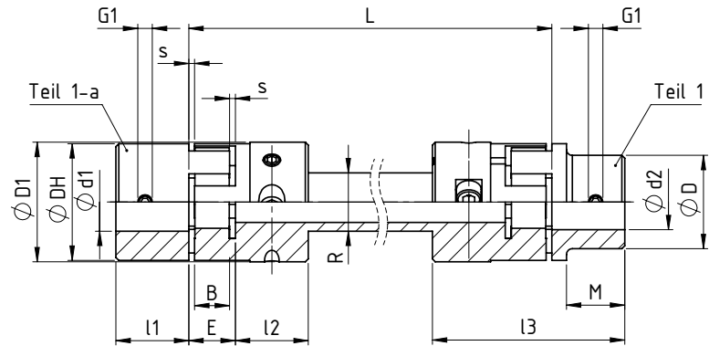
Passfedernut nach DIN 6885 keyway according to DIN 6885
