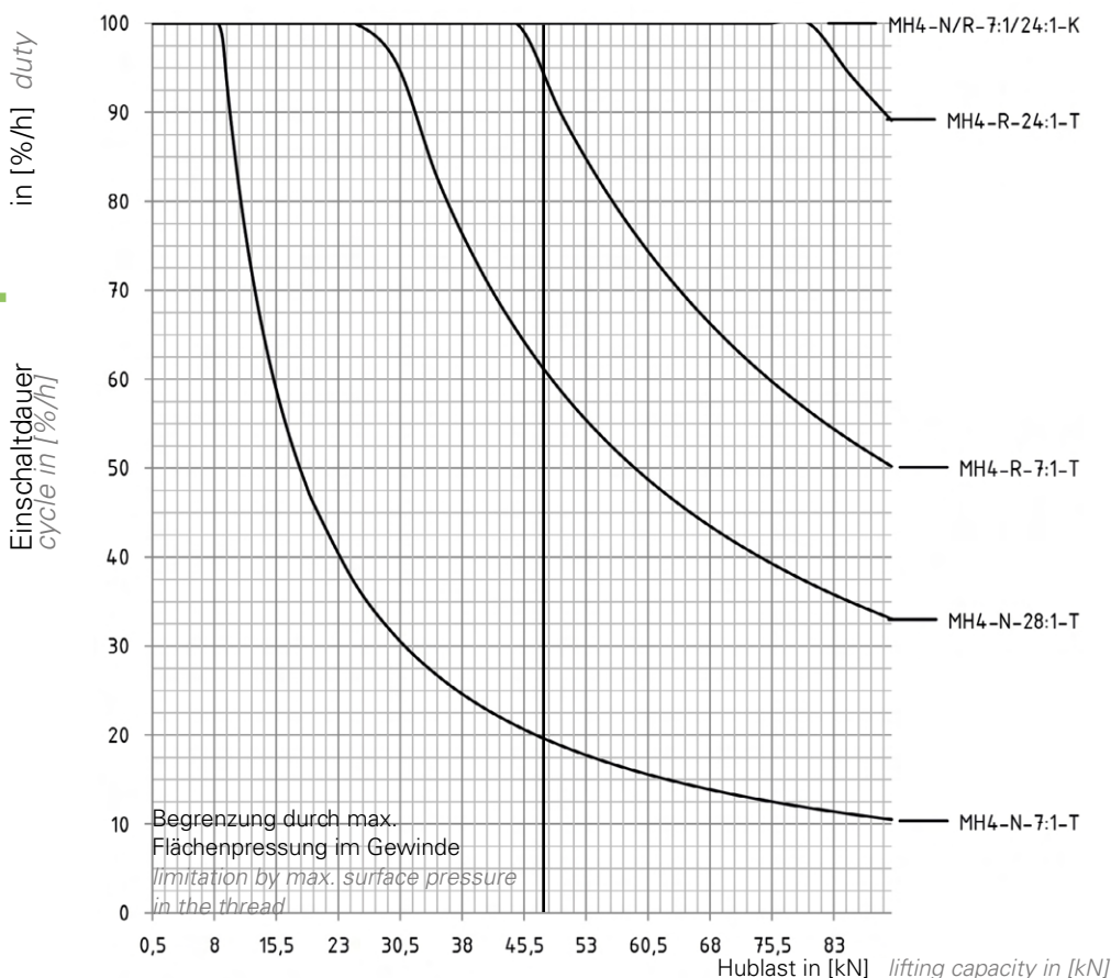
Einschaltdauerdiagramm MH4 duty cycle diagram MH4
