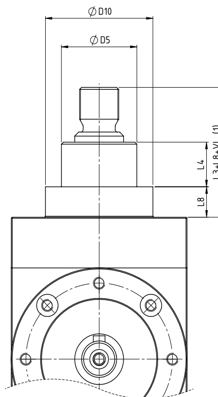
Darstellung für Ausführung mit erhöhtem Lagerdeckel. Illustration for version with raised bearing cover.
