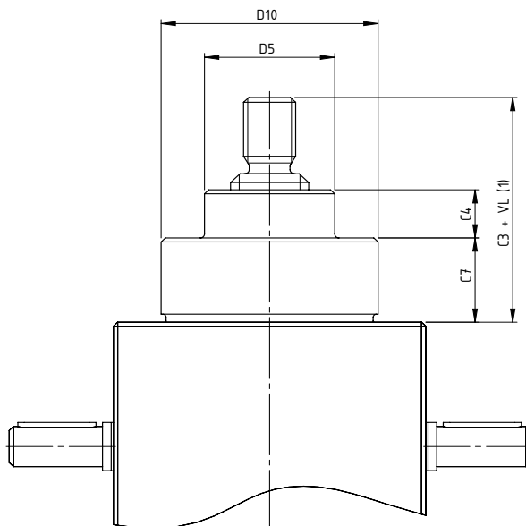
Darstellung für Ausführung mit erhöhtem Lagerdeckel. Illustration for version with raised bearing cover.
